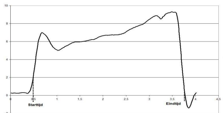
Figuur 3: Resultaat remvertragsingsmeting
