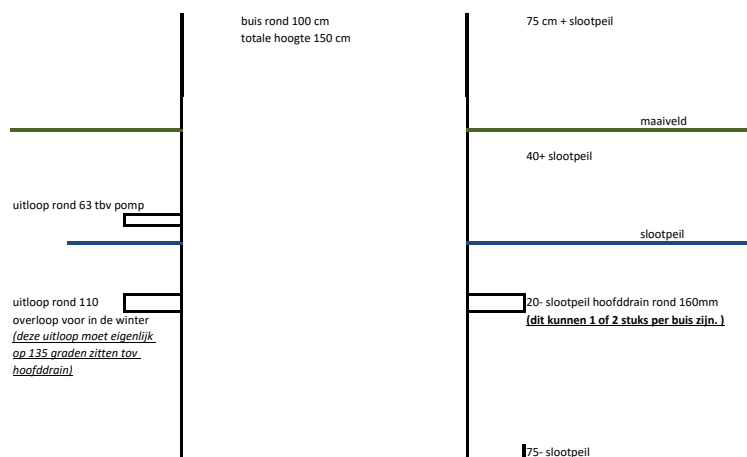
Afb 6: voorbeeld waterreservoir (regel- of pompput)
